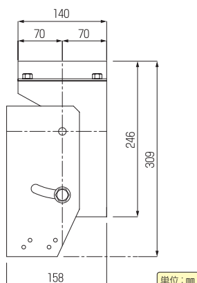
【側面図】
