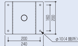
●天井ベース[平面]
