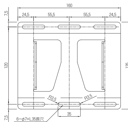
ベース金具寸法図
