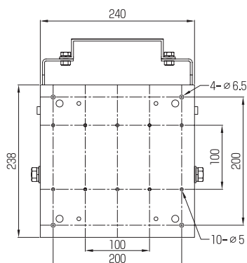
【正面図】
