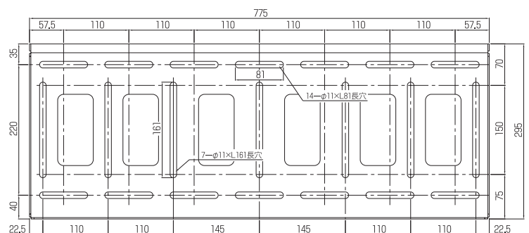
ベース金具寸法図
